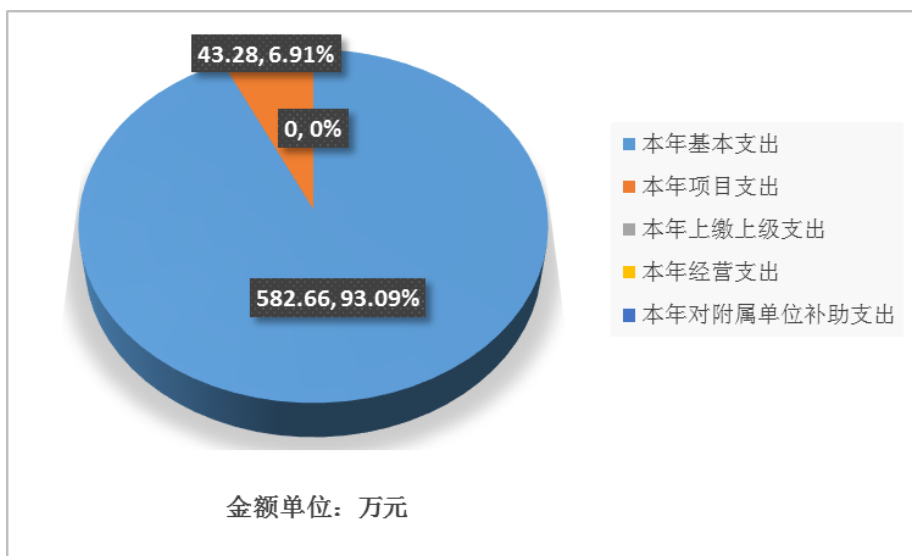
图 2. 支出决算图
